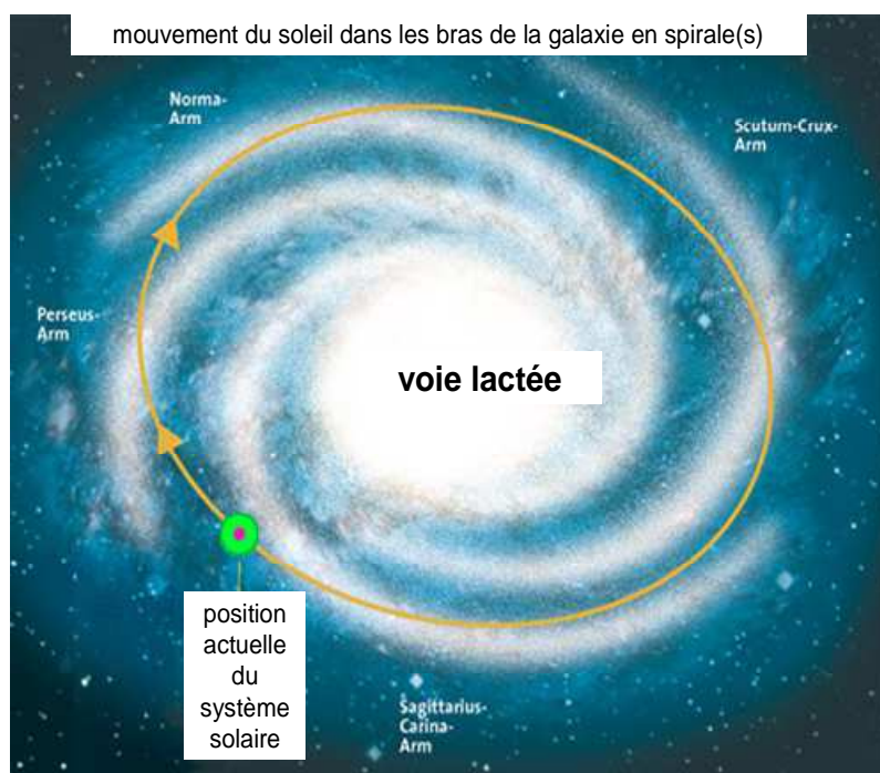
Figure 7-A Mouvement du système solaire dans la voie lactée (source BGR)
