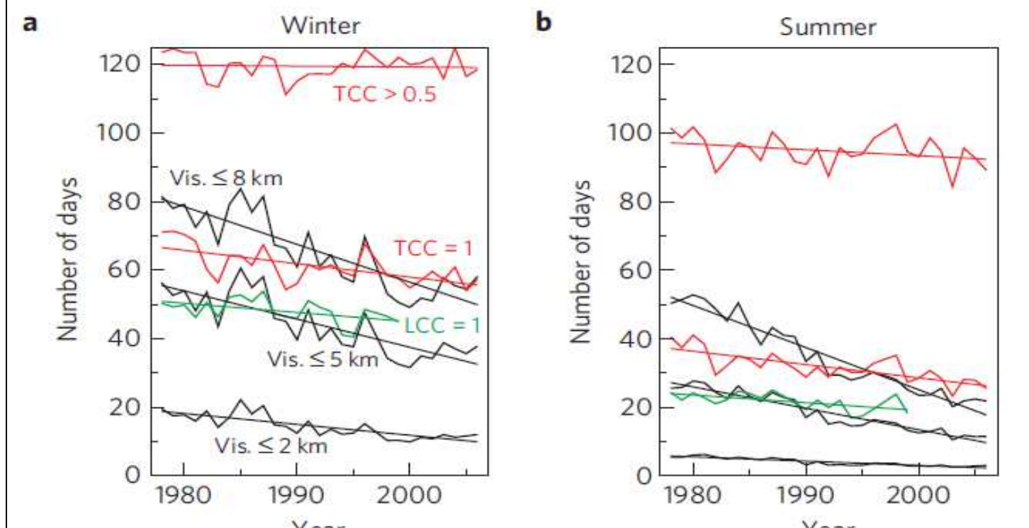
figure 19-E Europe occidentale 1978-2007: Nombre de jours avec une couverture nuageuse (TCC, Total Cloud Cover en rouge) supérieure à \frac{1}{2} et avec une couverture totale (TCC=1), nombre de jours avec une couverture de nuages bas (LCC, Low Cloud Cover en vert) totale (LCC=1) et nombre de jours avec une visibilité limitée à 2 km, 5 km et 8 km (R. Vautard et al. 2009)
