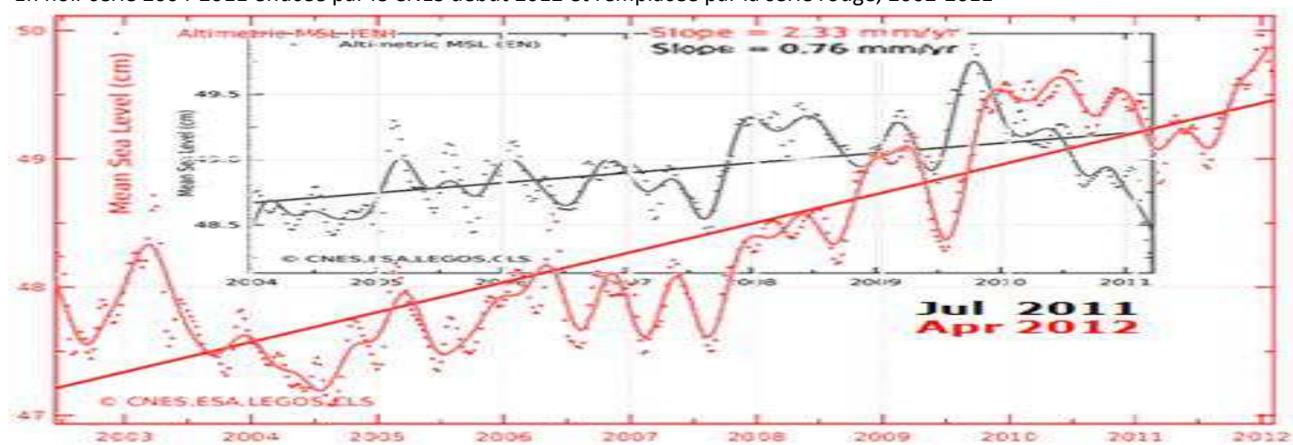
Figure 8-C Niveau moyen des mers Données initialement publiées du satellite ENVISAT et données "retraitées" En noir série 2004-2011 effacée par le CNES début 2012 et remplacée par la série rouge, 2002-2011
