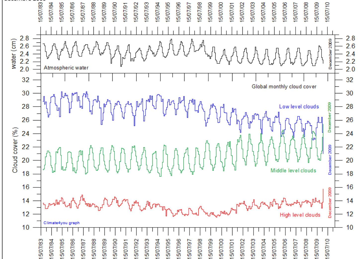
Figure 18-C Couverture nuageuse des trois types de nuages et contenu moyen de l'air en vapeur d'eau précipitable juillet 1983 à décembre 2009
