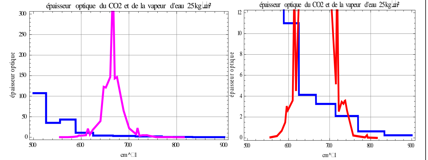
Figure 6-B zoom sur la raie du CO 2 et sur son pied en dessous de la tropopause.
