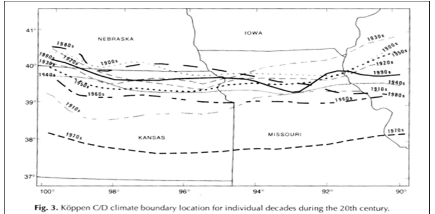
Figure 21-B Variations de la limite entre climats C et D de Köppen aux Etats Unis XXème siècle, par décennie, de 1900-1910 à 1990-2000
