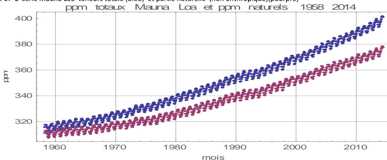
Figure 17-C série Mauna Loa teneurs totale (bleu) et partie naturelle (non anthropique)(pourpre)
