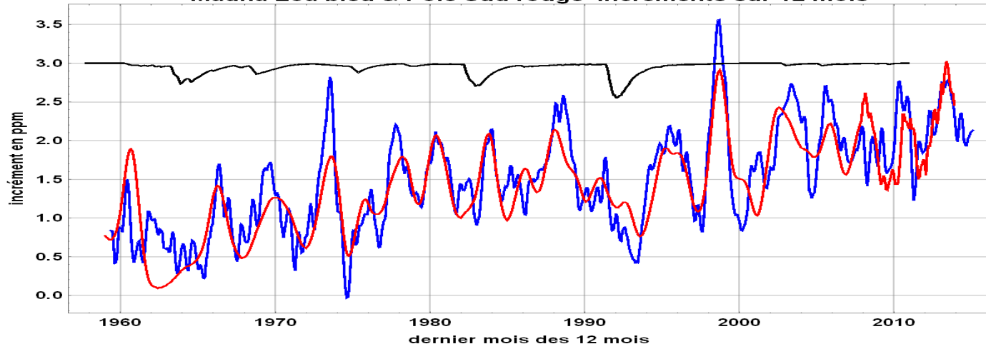
Mauna Loa bleu & Pôle Sud rouge incréments sur 12 mois
