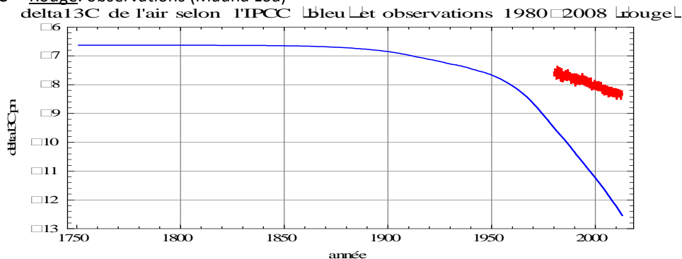
Figure 4-C Bleu: \delta^{13}\text{C} de l'air calculé selon la formule de Berne de IPCC (AR4 page 213) en prenant \{-6,5 \text{ pm} \& 277 \text{ ppm}\} comme valeurs "préindustrielles" et en supposant que ce sont les molécules de \text{CO}_2 anthropique qui restent dans l'air comme le laisse entendre le GIEC Rouge: observations (Mauna Loa)
