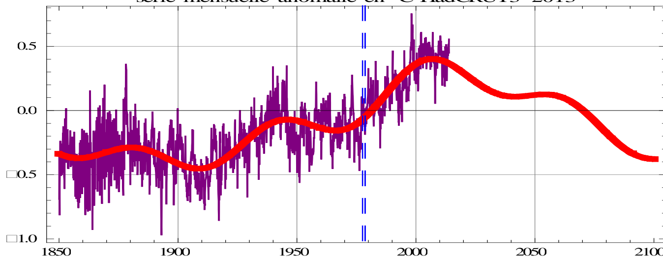
série mensuelle anomalie en ^\circ\text{C} HadCRUT3 2013
