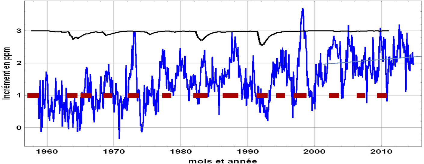
MaunaLoa incréments d[\text{CO}_2]/dt pour dt=12 mois centrés
