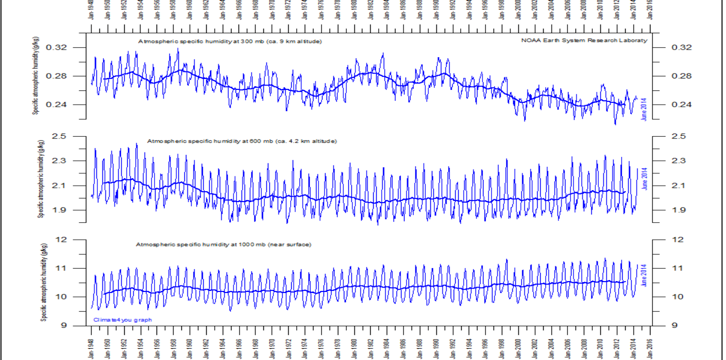
Figure 10-B quantité de vapeur d'eau à 300 mbar (9 km), 600 mbar (4.2 km) et 1000 mbar, Janv. 1948 à Juin 2014
