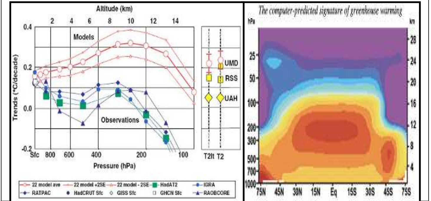
Figure 9-B Comparaison des observations (à gauche) et des prétendus modèles (selon IPCC 2007) qui eux montrent le hot spot près de la tropopause entre 400 mbar et 200 mbar (ou hPa), en degré/dix ans Multiplier par dix pour passer en degrés par siècle
