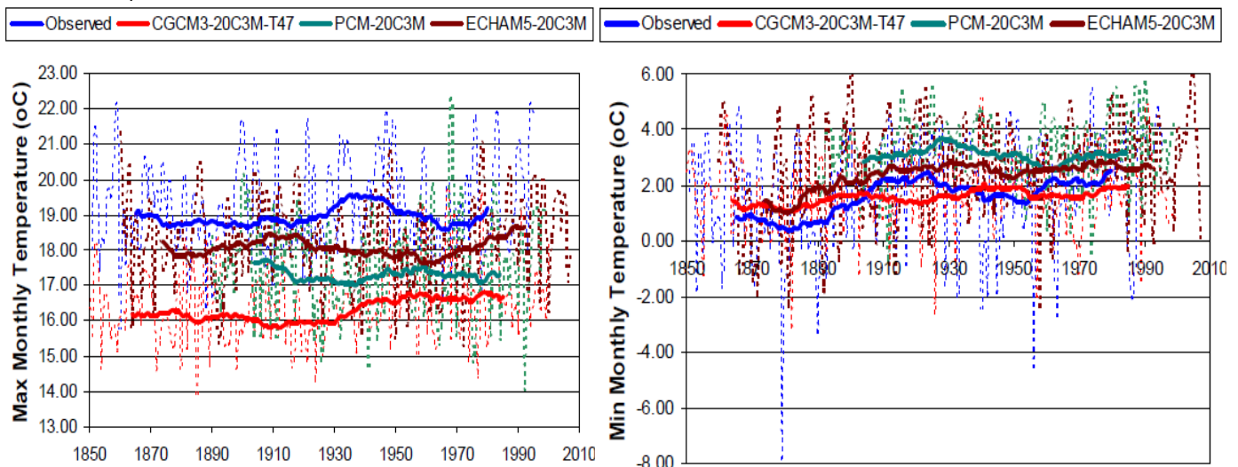
Figure 20-C Comparaison des observations et des rétro-prédictions des prétendus modèles: Paris, France températures des mois le plus chaud et le plus froid 1850-2005. Les observations sont en bleu
