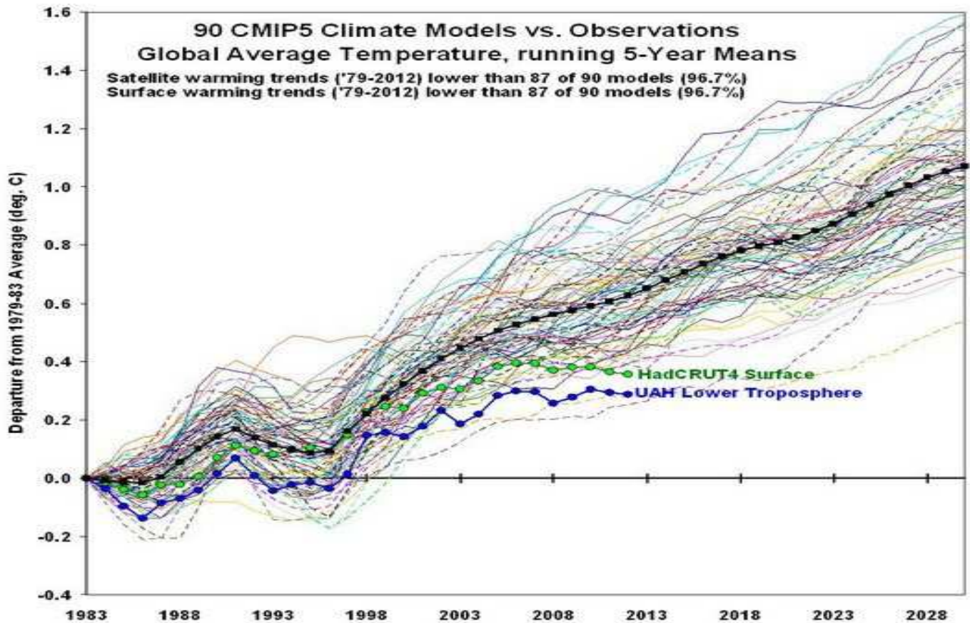
Figure 20-B Températures de surface en moyenne mondiale: comparaison de 90 modèles CMIP (pour le rapport IPCC 2013) et des séries HadCRUT4 (températures de surface) et UAH MSU (basse troposphère) Noter le saut observé de 0,2°C ou 0,3°C lors du grand El Niño de 1997-98. Les modèles ont été décalés pour passer tous par le même point {0°C, 1983}
