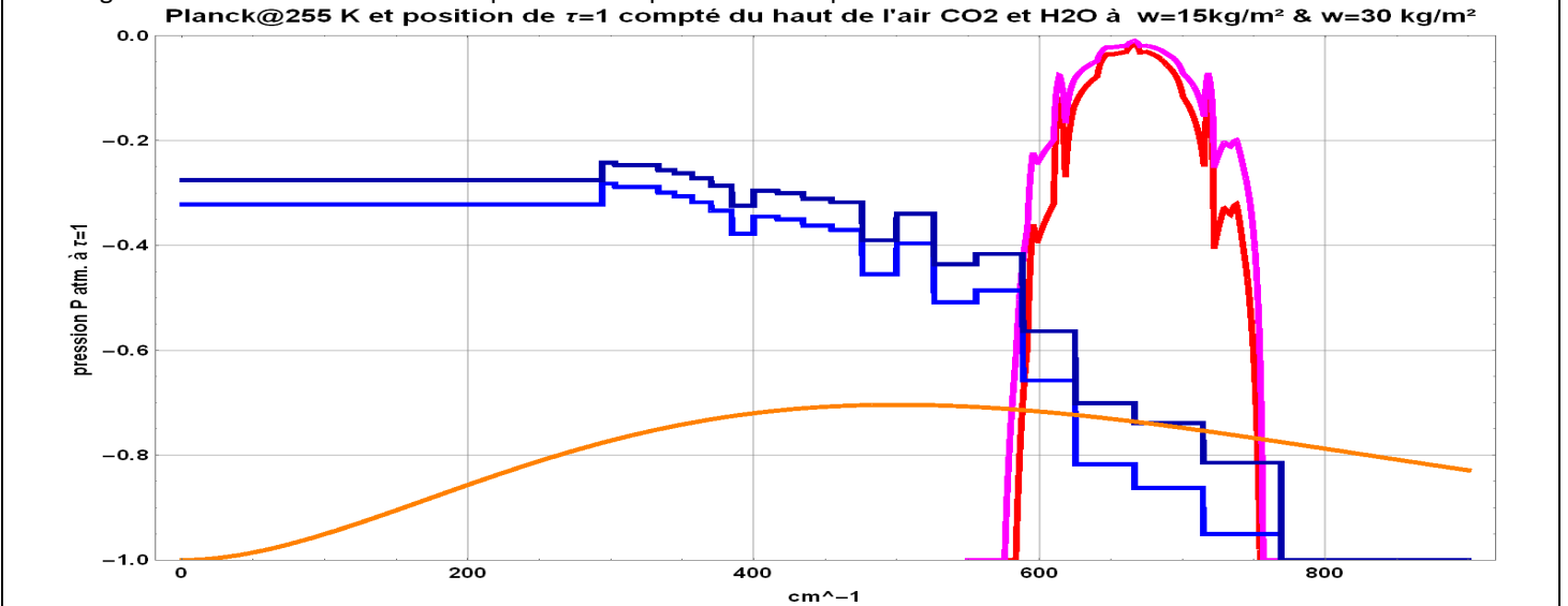
Figure 6-E) Pression en atmosphère de la couche au-dessus de laquelle 80% des photons rayonnés vers le cosmos En bleu pour la vapeur d'eau, en rouge et magenta pour le dioxyde de carbone aux teneurs actuelles et après "doublement" En orange allure de la fonction de Planck pour une température de corps noir de 255 K
