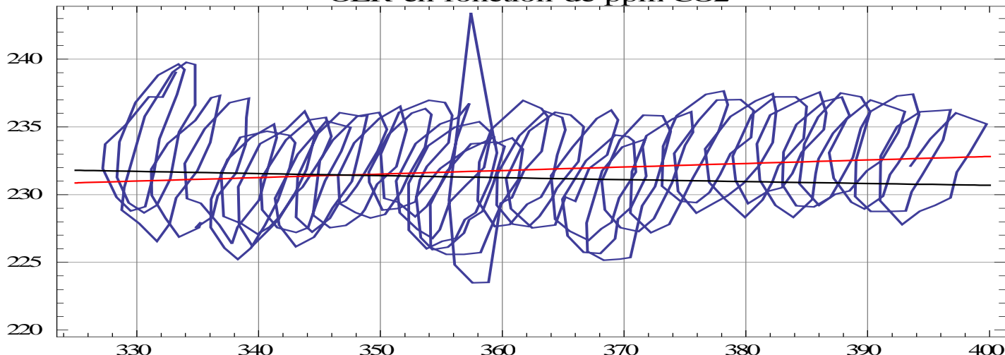
OLR en fonction de ppm CO 2
