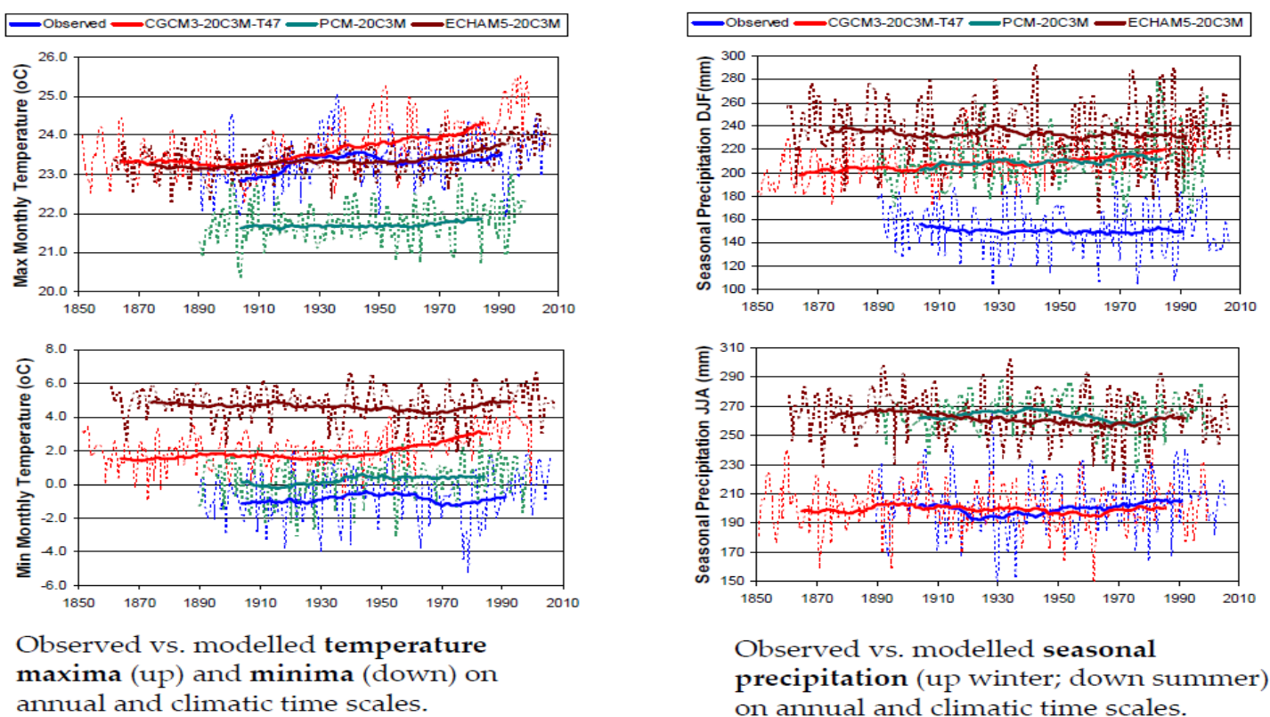
Figure 20-D Comparaison des observations et des prétendus "modèles": Etats-Unis, températures des mois le plus chaud et le plus froid 1850-2005 et précipitations en hiver et en été. Les observations sont en bleu.
