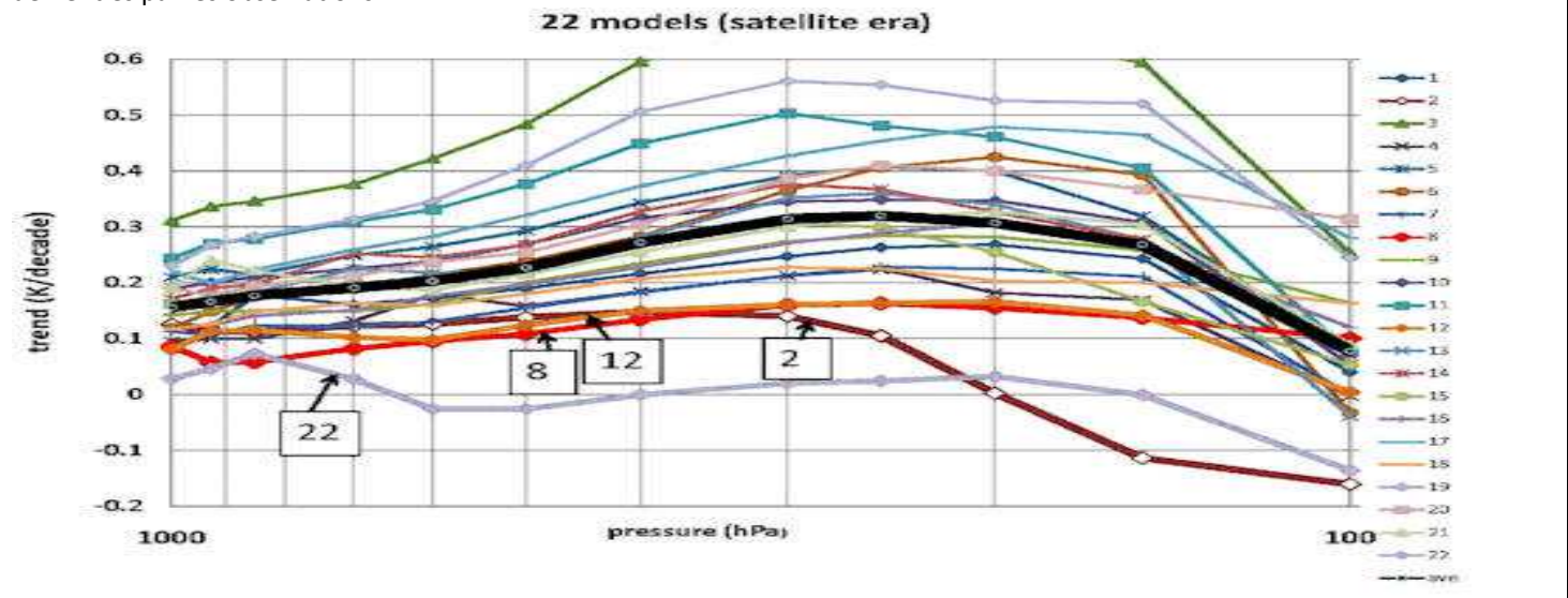
Figure 9-C Comparaison des tendances en °C/dix ans selon 22 prétendus modèles entre la surface et 100 hPa 1979-2005 le détail des modèles est donné à la figure ci-dessous; comme montré plus haut ces élucubrations assistées par ordinateur sont démenties par les observations
