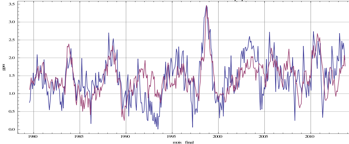
Mauna Loa incréments moins effet anthropique
