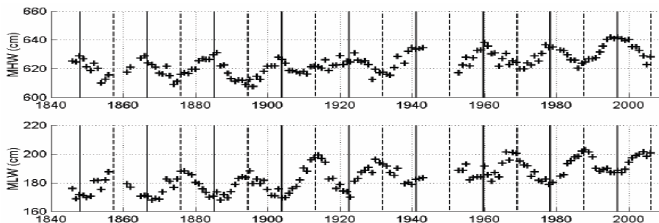
Fig. 1.5 – Niveau moyen annuel de la pleine mer (MHW) et niveau moyen annuel de la basse mer (MLW) à Brest entre 1846 et 2007. Les lignes verticales continues et les lignes verticales en pointillés correspondent au moment du minimum (respectivement du maximum) de la déclinaison de la Lune. Valeurs des minimums et maximums de la déclinaison de la Lune d'après Pugh (2004).
