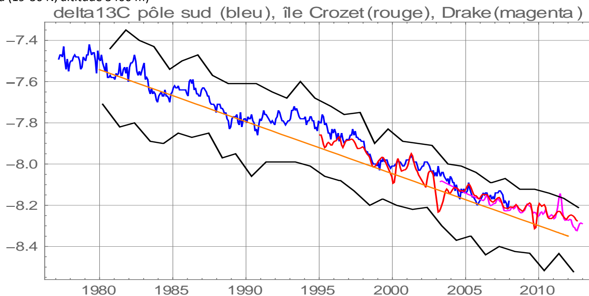
Figure 3-A Moyennes annuelles des observations du delta 13 C (en pour mille, pm) mois par mois au pôle sud (en bleu), à l'île Crozet (en rouge), au passage de Drake (en magenta) et enveloppe (minima et maxima annuels) des observations à l'observatoire du Mauna Loa (19°30'N, altitude 3400 m)
