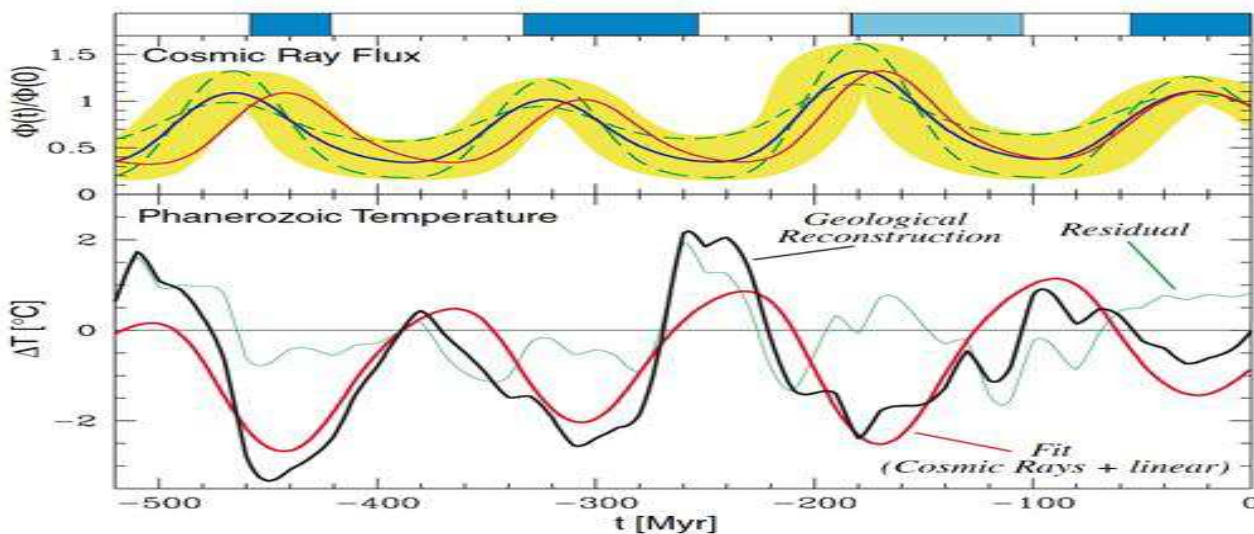
Figure 7-B Comparaison des flux de rayons cosmiques galactiques et des températures en zone intertropicale
