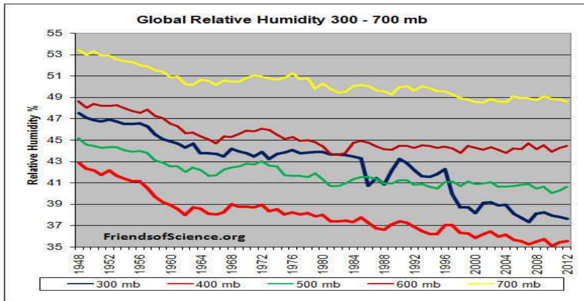
Figure 10-C Variations de l'humidité relative depuis 1948 selon les observations des ballons-sondes à 700 mbar, 600 mbar, 500 mbar, 400 mbar et 300 mbar. (voir aussi http://www.esrl.noaa.gov/psd/cgi-bin/data/timeseries/timeseries1.pl qui part des réanalyses)
